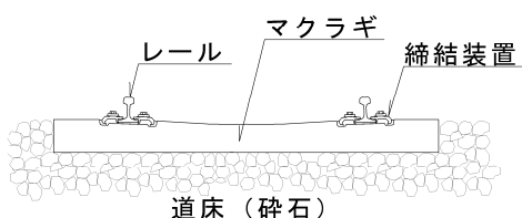
線路の標準的な横断面図
