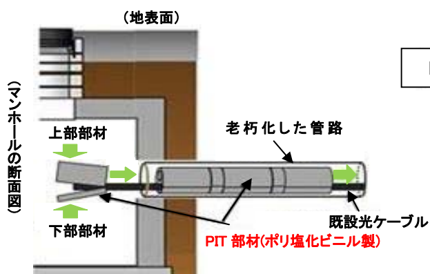
PIT 部材(ポリ塩化ビニル製)
