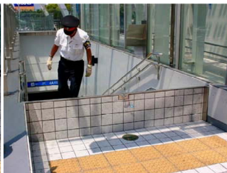
▲立上式止水板（立ち上げ時）
